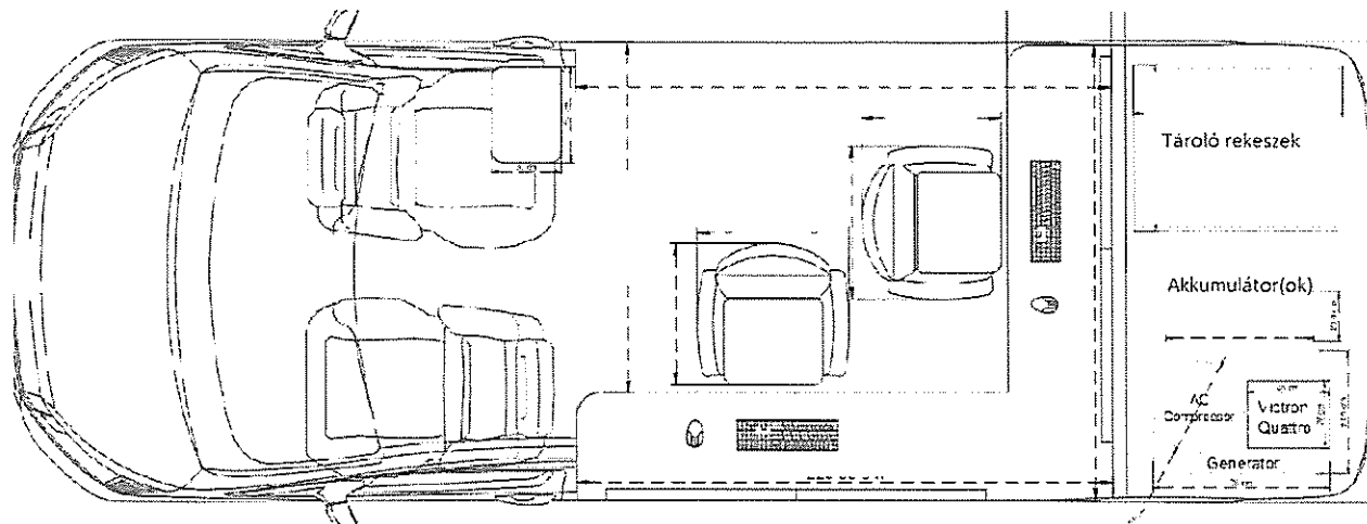
1. ábra. A jármű belső kialakításának terve. A beépítésre kerülő eszközök, felszerelési tárgyak tényleges elhelyezése opcionális, azok az ábrától eltérően (akár a jármű külső felületén) is elhelyezhetők, amennyiben a műszaki leírás egyéb feltételeit teljesítik. Az ábrával ellentétben a vezető fülke jobb első ülésének nem kell forgathatónak lennie, a gyári kivitelezés elfogadható.
